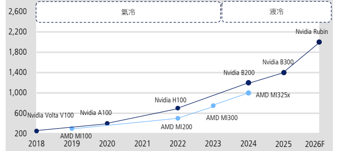
圖 56：GPU 散熱設計功耗(TDP)增長，將逐步帶動液冷散熱之需求
